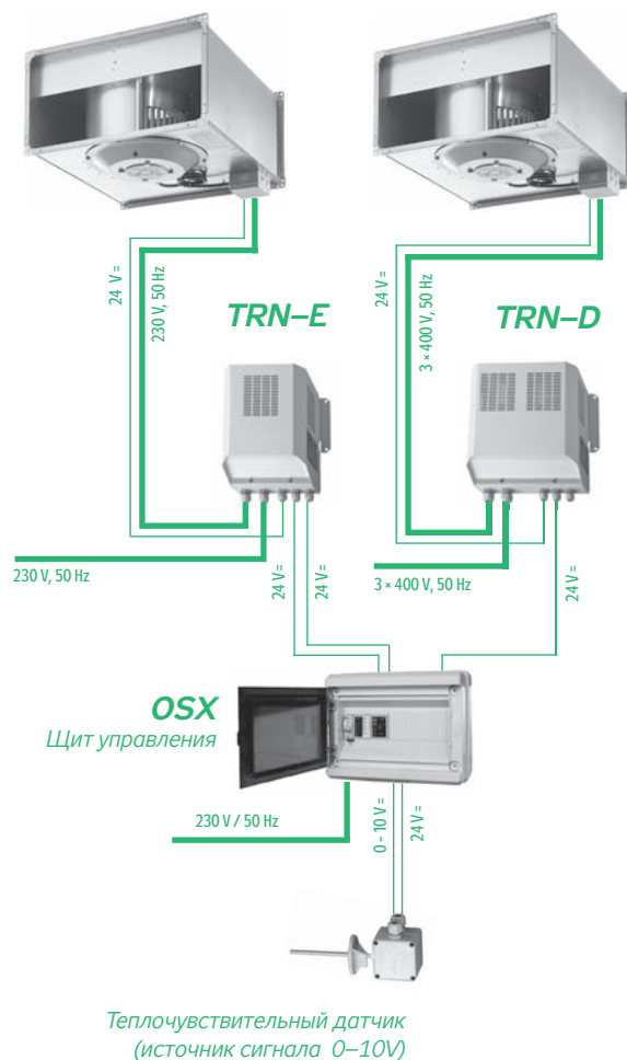
РИС. 11 – ПОДКЛЮЧЕНИЕ ВЕНТИЛЯТОРА
