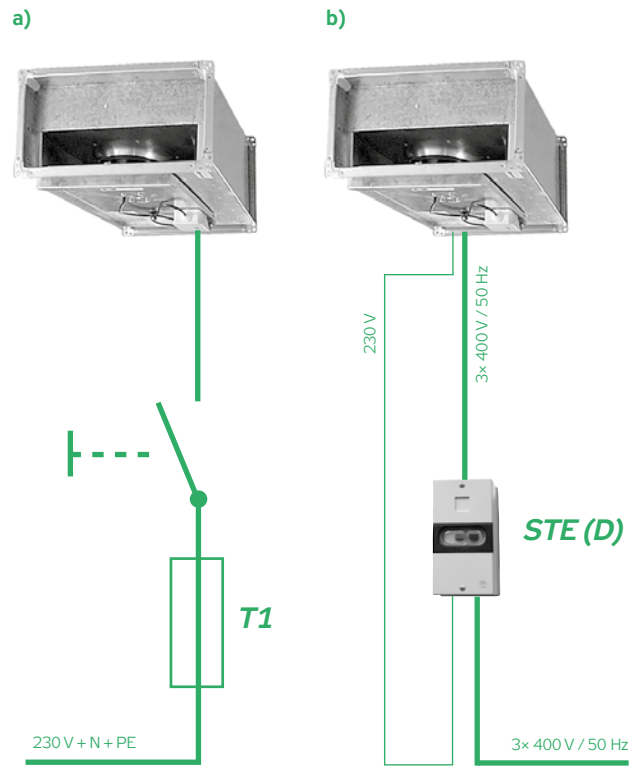
РИС. 5 – ПОДКЛЮЧЕНИЕ ВЕНТИЛЯТОРА
