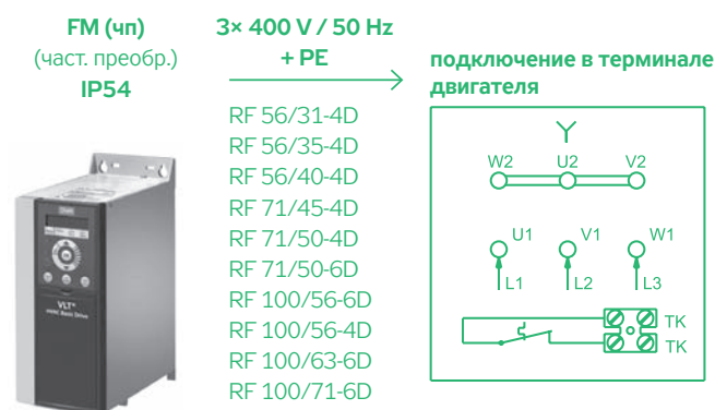
РИС.4 – ВКЛЮЧЕНИЕ Y/Δ НА КЛЕММНИКЕ ТРЕХФАЗНОГО ДВИГАТЕЛЯ С ЧАСТОТНЫМ ПРЕОБРАЗОВАТЕЛЕМ, ЗАЩИТА IP 54 (RFFMIMXXXX50)
