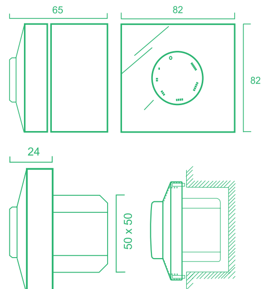
РИС. 39 – РАЗМЕРЫ ОРР (IP 54)
