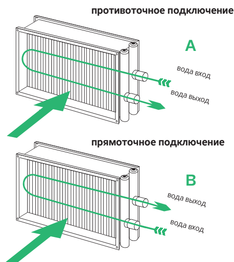
РИС. 11 – ПОДКЛЮЧЕНИЕ ОБОГРЕВАТЕЛЯ
