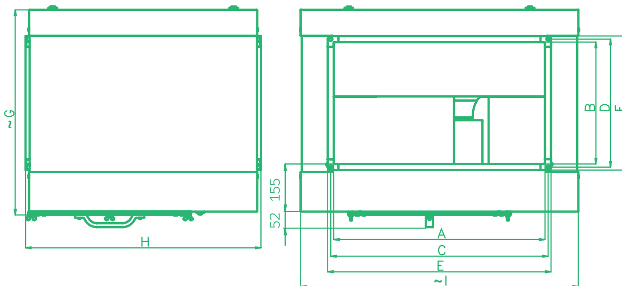
РИС. 4 – ОБОЗНАЧЕНИЕ РАЗМЕРОВ
