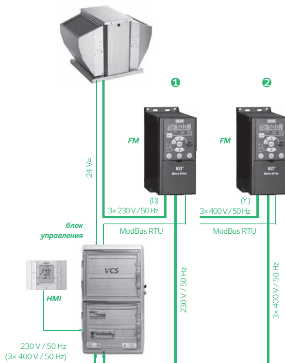
РИС.12 – ПОДКЛЮЧЕНИЕ ВЕНТИЛЯТОРА
