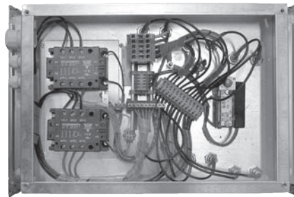
EOSX... / 22 - 45, EOSX... / 12 - 45 (содержат два или три 3-фазных пускателя SSR). Вид внутри электрощита обогревателя EOSX 70-40/30.
