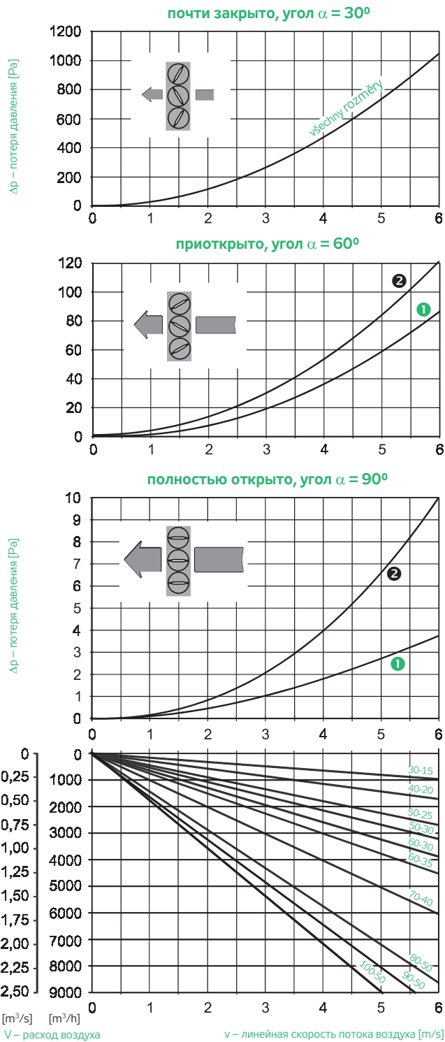
ГРАФИК 1 – ПОТЕРЯ ДАВЛЕНИЯ РЕГУЛИРУЮЩИХ И ОТСЕКАЮЩИХ ЗАСЛОНКИ LKR, LKS, LKSX, LKSF
