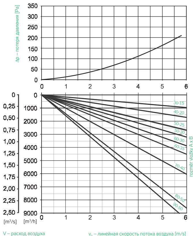
ГРАФИК 1 – ПОТЕРЯ ДАВЛЕНИЯ ФИЛЬТРОВ VFК В НЕЗАГРЯЗНЕННОМ СОСТОЯНИИ
