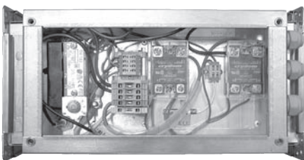
EOS... / 3, (содержит два 1-фазных пускателя SSR) Вид внутри электрощита обогревателя EOS 30-15/3 при открытии крышки пускателей SSR.
