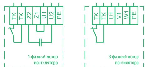
РИС. 4 – СХЕМЫ ПОДКЛЮЧЕНИЯ
