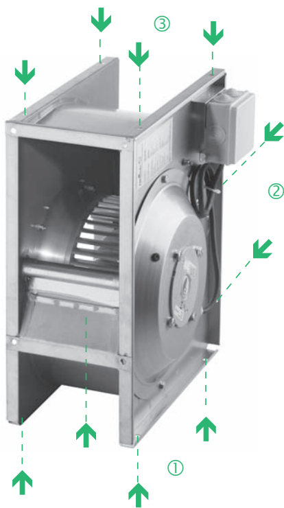
РИС. 3 – МОНТАЖНЫЕ ОТВЕРСТИЯ
