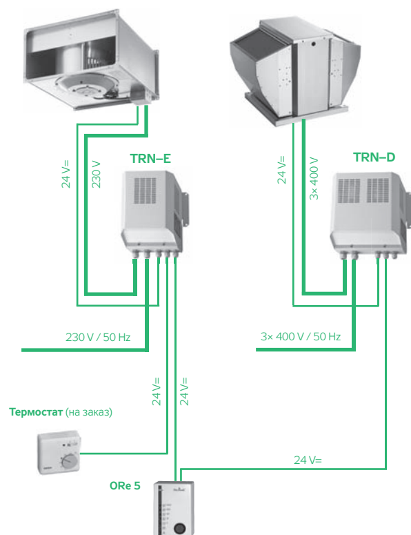
РИС. 22 – ПОДКЛЮЧЕНИЕ РЕГУЛЯТОРОВ
