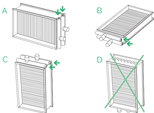
РИС. 8 – ПОЛОЖЕНИЯ ОБОГРЕВАТЕЛЯ
