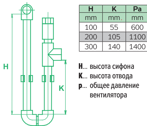
РИС. 5 – ОТВОД КОНДЕНСАТА
