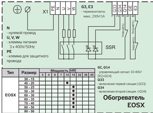
РИС. 21 – СХЕМА ПОДКЛЮЧЕНИЯ ОБОГРЕВ. EOSX
