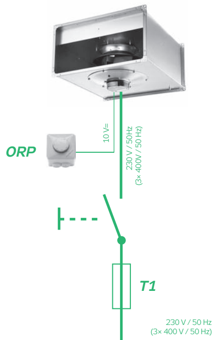
РИС. 7 – ПОДКЛЮЧЕНИЕ ВЕНТИЛЯТОРА
