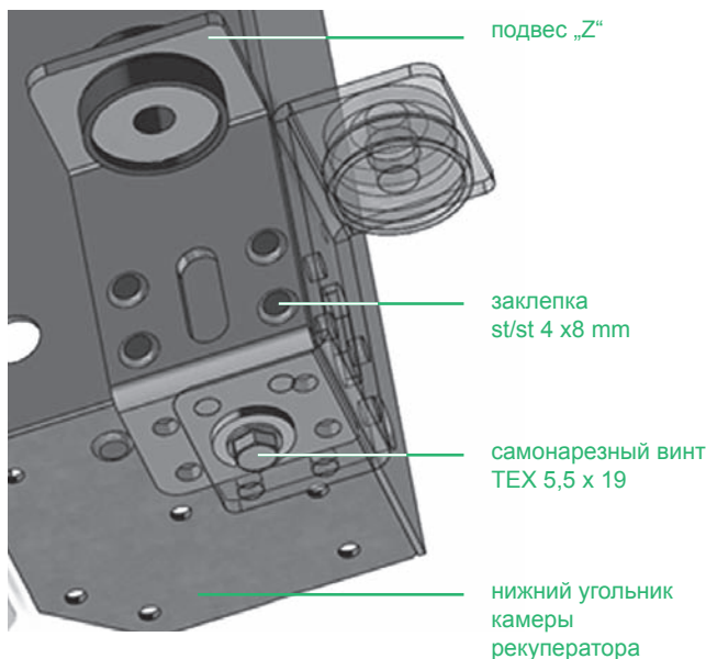
РИСУНОК 12 – МОНТАЖ НА ПОДВЕС Z
