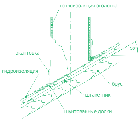
РИС.19 – ПОДСТАВКА ДЛЯ СКАТНОЙ (НАКЛОННОЙ) КРЫШИ
