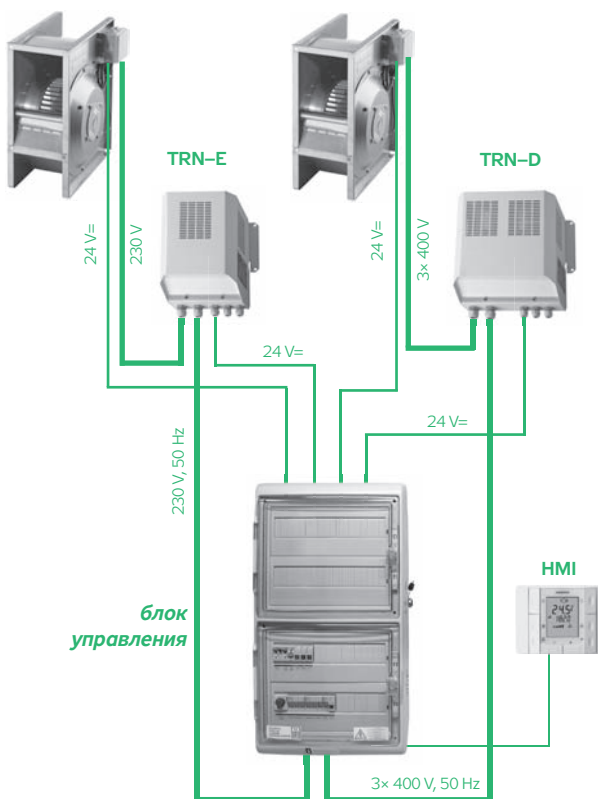
РИС. 8 – ПОДКЛЮЧЕНИЕ ВЕНТИЛЯТОРА
