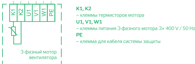
РИС. 10 – СХЕМЫ ПОДКЛЮЧЕНИЯ
