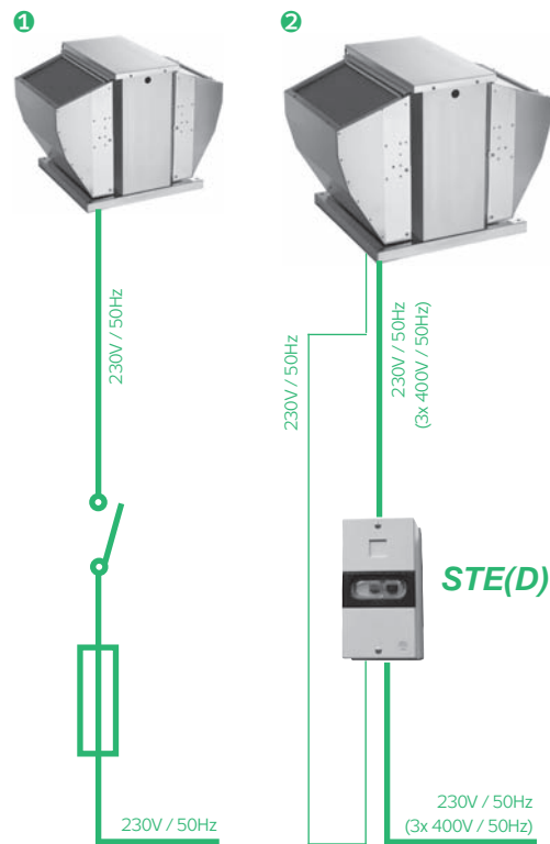
РИС.6 – ПОДКЛЮЧЕНИЕ ВЕНТИЛЯТОРА
