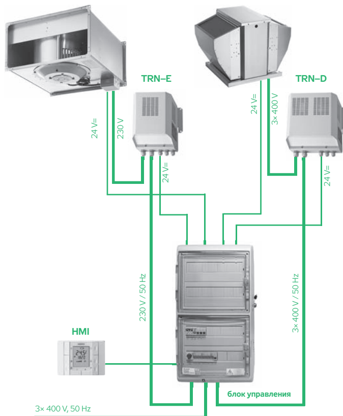
РИС. 23 – ПОДКЛЮЧЕНИЕ РЕГУЛЯТОРОВ
