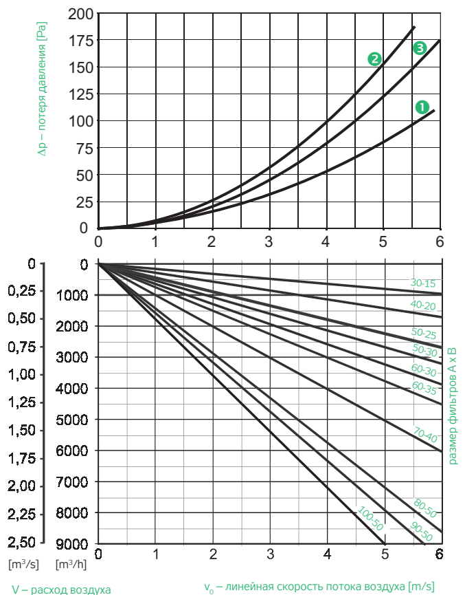
ГРАФИК 1 – ПОТЕРЯ ДАВЛЕНИЯ ФИЛЬТРОВ KF5 В НЕЗАГРЯЗНЕННОМ СОСТОЯНИИ
