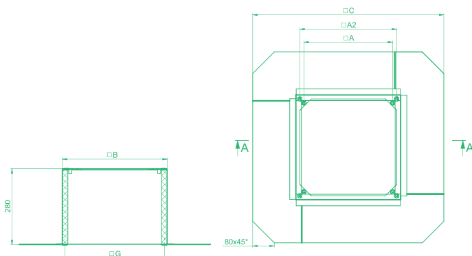
РИС.14 – РАЗМЕРЫ ПОДСТАВОК NK
