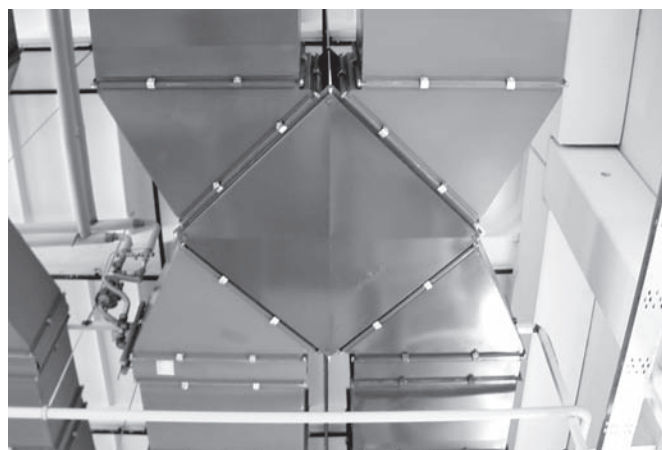
РИС. 13 – СОЕДИНЕНИЕ ПОСЕРЕДИНЕ СКОБОЙ
