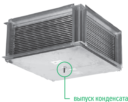
РИС. 5 – PVC ВЫПУСК
