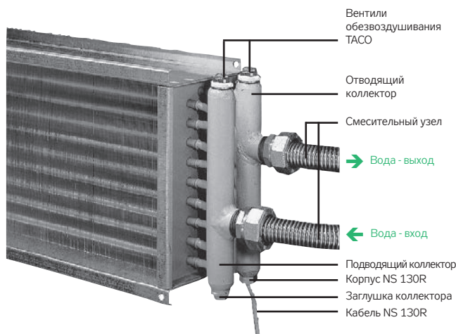
РИС. 10 – УСТАНОВКА ВЕНТИЛЕЙ ТАСО
