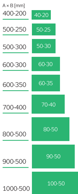
РИС. 1 – ТИПОРАЗМЕРЫ
