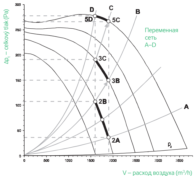
РИС. 4 – РАБОЧИЕ СОСТОЯНИЯ СИСТЕМЫ
