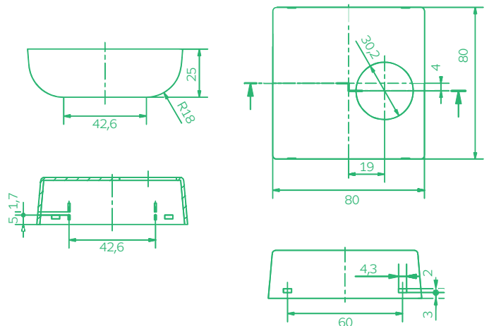
РИС. 37 – РАЗМЕРЫ ОРР (IP 40)
