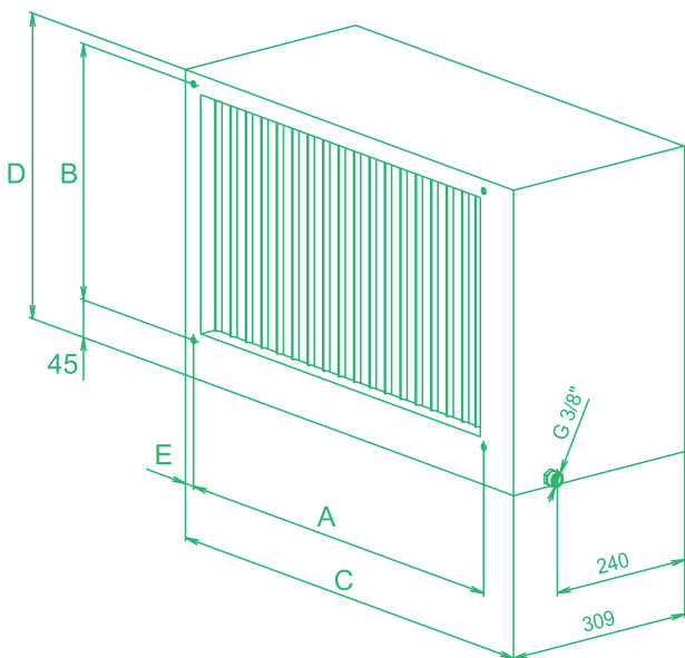
РИСУНОК 1 – ТИПОРАЗМЕРЫ КАПЛЕУЛОВИТЕЛЯ
