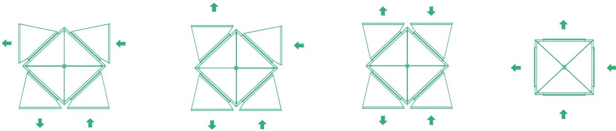
РИС. 6 – ВАРИАНТЫ РАЗМЕЩЕНИЯ РЕКУПЕРАТОРА В КАНАЛЕ В СООТВЕТСТВИИ С ОРИЕНТИРОВКОЙ КОЛЕН OBL ... /45
