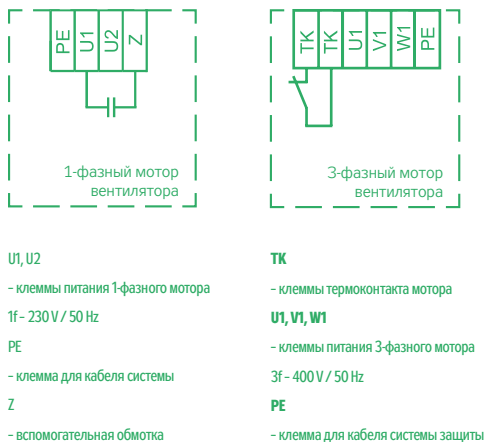
РИС. 4 – СХЕМЫ ПОДКЛЮЧЕНИЯ
