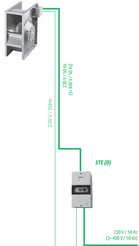
РИС. 5 – ПОДКЛЮЧЕНИЕ ВЕНТИЛЯТОРА
