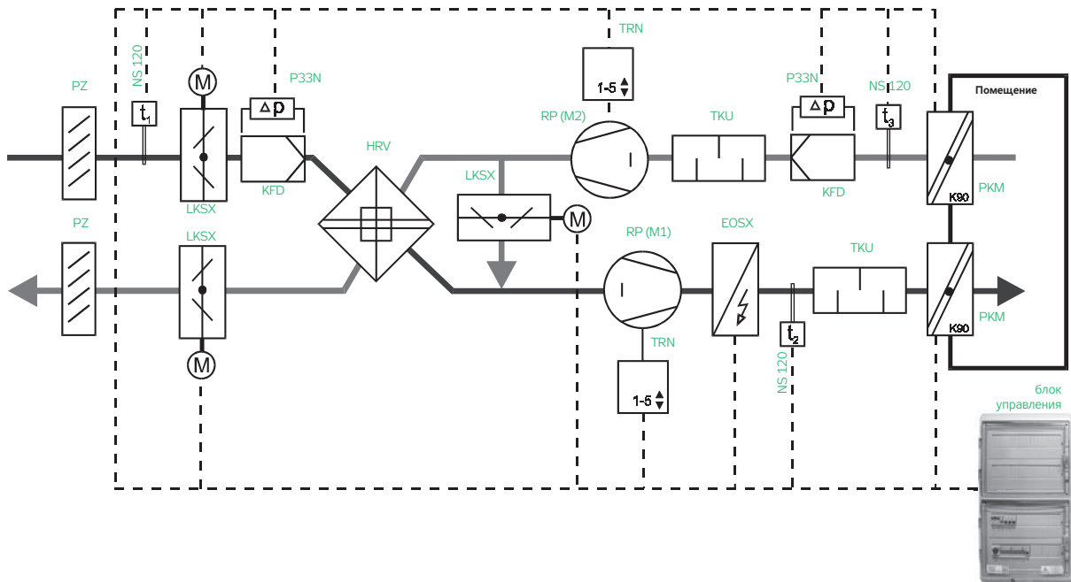
РИС. 15 – РЕКУПЕРАТОР С БАЙПАСОМ
