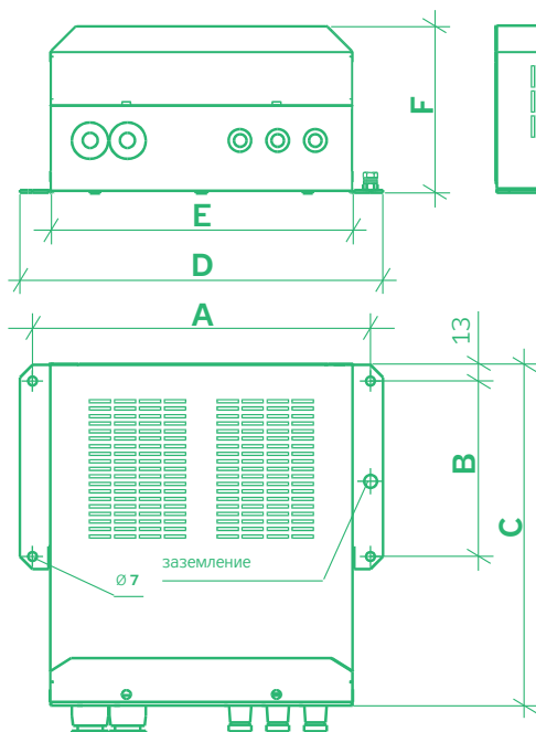
РИС. 15 – РАЗМЕРЫ И ВЕС РЕГУЛЯТОРОВ TRN
