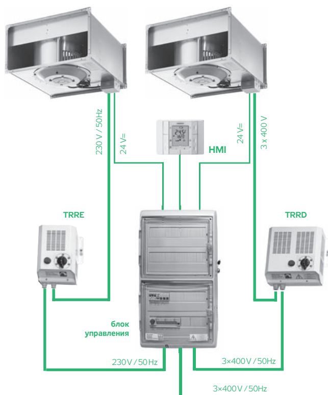
РИС. 35 – ПОДКЛЮЧЕНИЕ РЕГУЛЯТОРОВ
