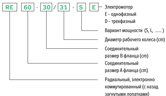
РИС. 3 – ТИПОВОЙ КЛЮЧ ДЛЯ ОБОЗНАЧЕНИЯ ВЕНТИЛЯТОРОВ
