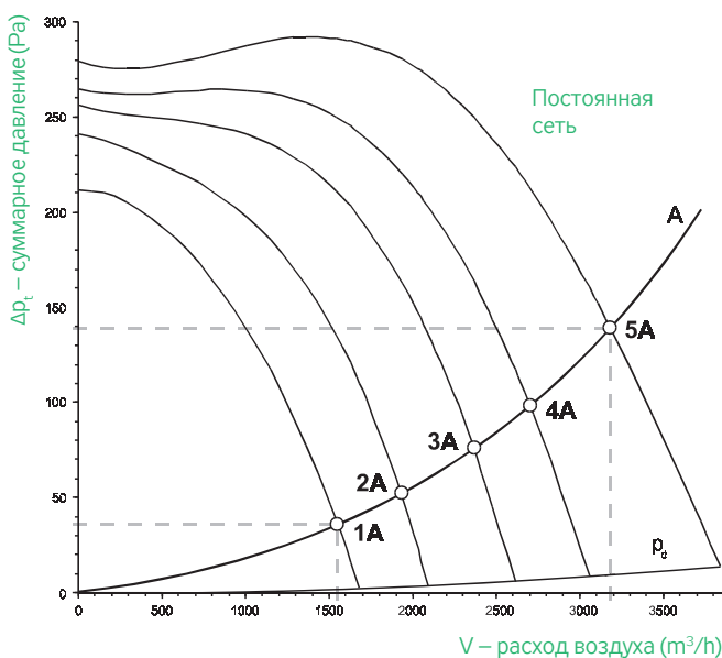
РИС. 1 – МАКС.РАСХОД ВОЗДУХА
