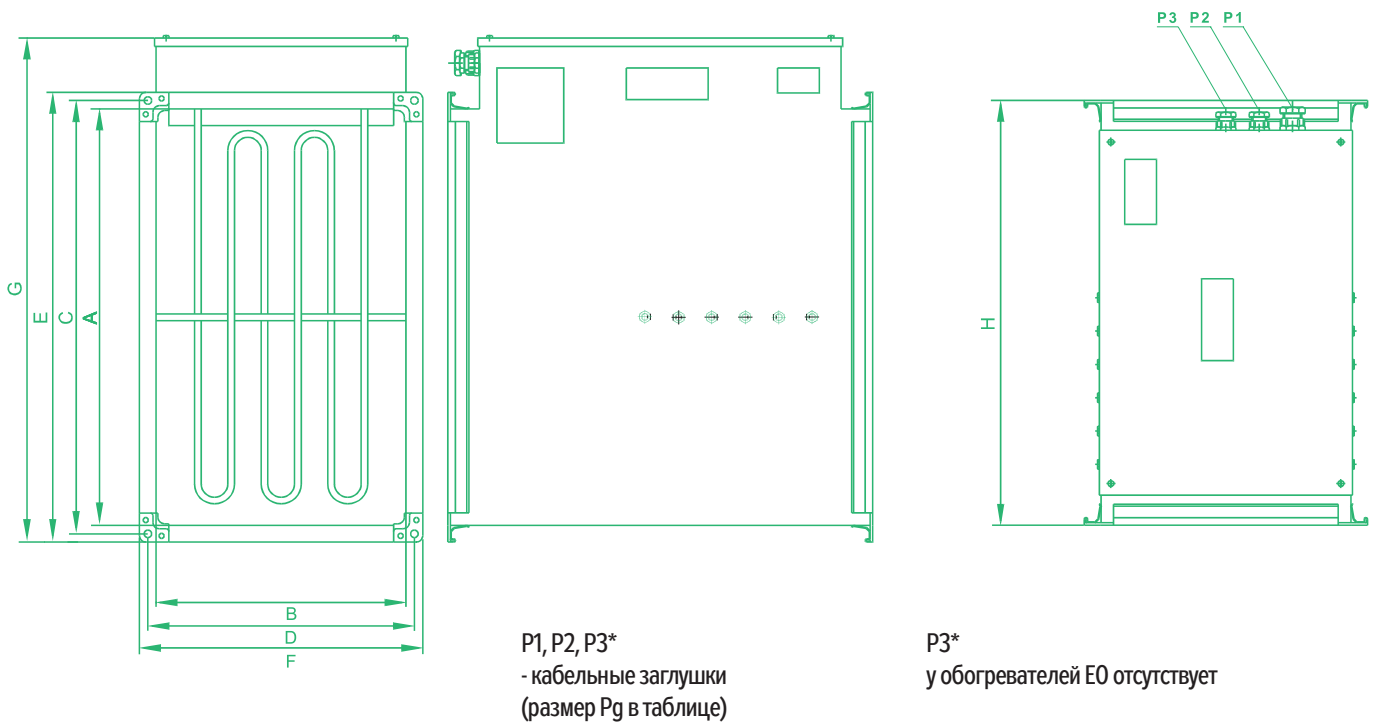
РИС. 3 - РАЗМЕРЫ И ВЕС
