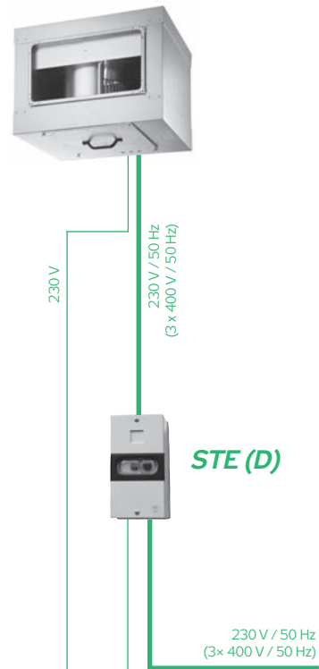
РИС. 6 – ПОДКЛЮЧЕНИЕ ВЕНТИЛЯТОРА
