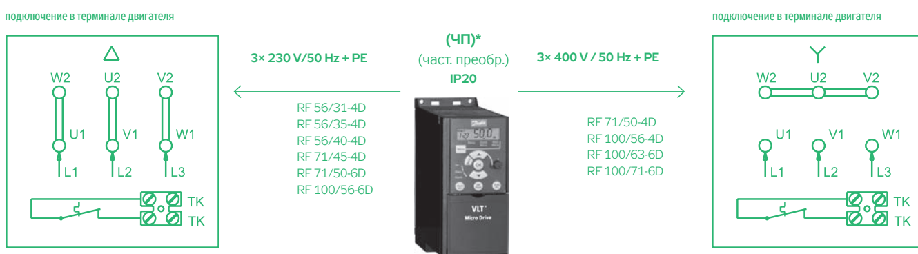
РИС.3 – ВКЛЮЧЕНИЕ Y/Δ НА КЛЕММНИКЕ ТРЕХФАЗНОГО ДВИГАТЕЛЯ С ЧАСТОТНЫМ ПРЕОБРАЗОВАТЕЛЕМ, ЗАЩИТА IP 21 (RFFMIMXXXX20)
