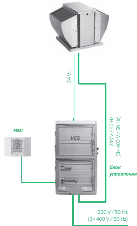
РИС.10 – ПОДКЛЮЧЕНИЕ ВЕНТИЛЯТОРА
