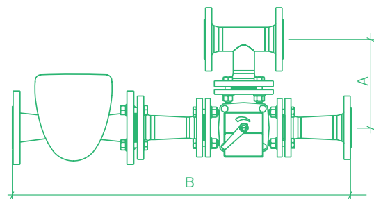
РИС. 4А – ОСНОВНАЯ КОМПОНОВКА
