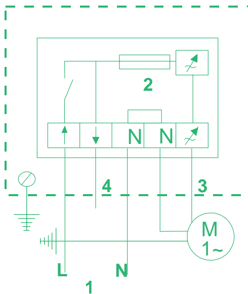
РИС. 48 – ПОДКЛЮЧЕНИЕ ВЕНТИЛЯТОРА
