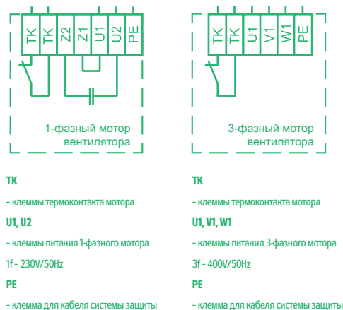
РИС. 5 – СХЕМЫ ПОДКЛЮЧЕНИЯ
