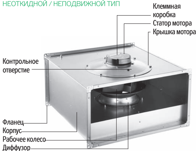
РИС. 4 – СОСТАВ ВЕНТИЛЯТОРА RE НЕОТКИДНОЙ / НЕПОДВИЖНОЙ ТИП
