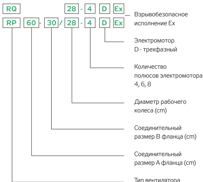
РИС. 3 – ТИПОВОЙ КЛЮЧ ДЛЯ ОБОЗНАЧЕНИЯ
