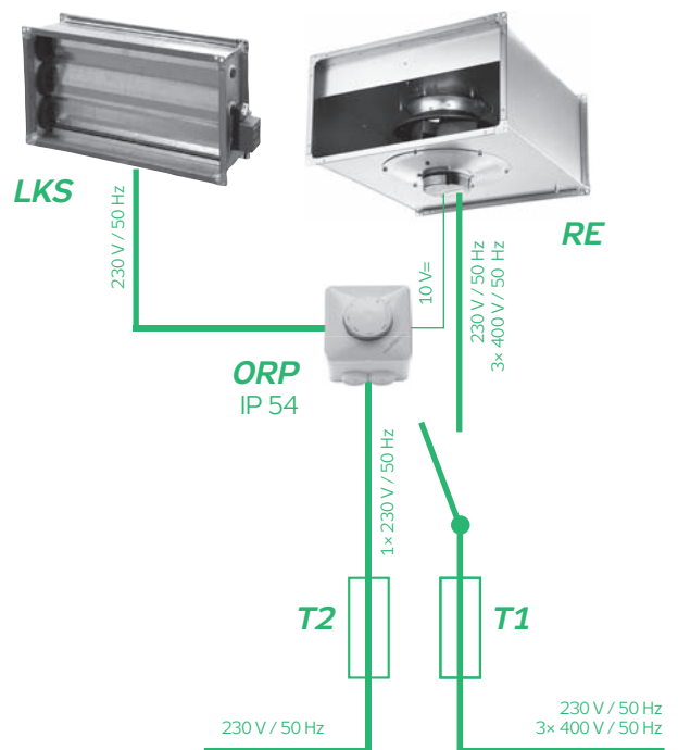
РИС. 22 – ПОДКЛЮЧЕНИЕ КОМАНДОАППАРАТА
