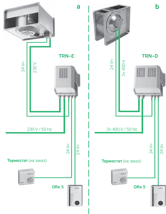
РИС. 21 – ПОДКЛЮЧЕНИЕ РЕГУЛЯТОРОВ
