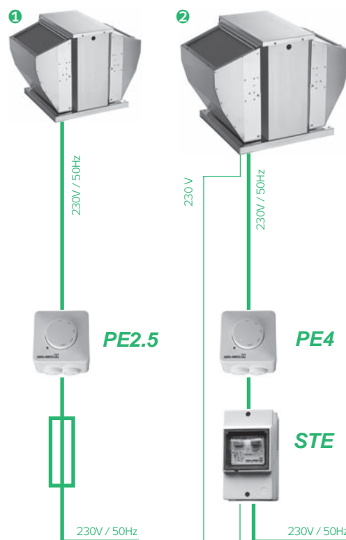
РИС.7 – ПОДКЛЮЧЕНИЕ ВЕНТИЛЯТОРА
