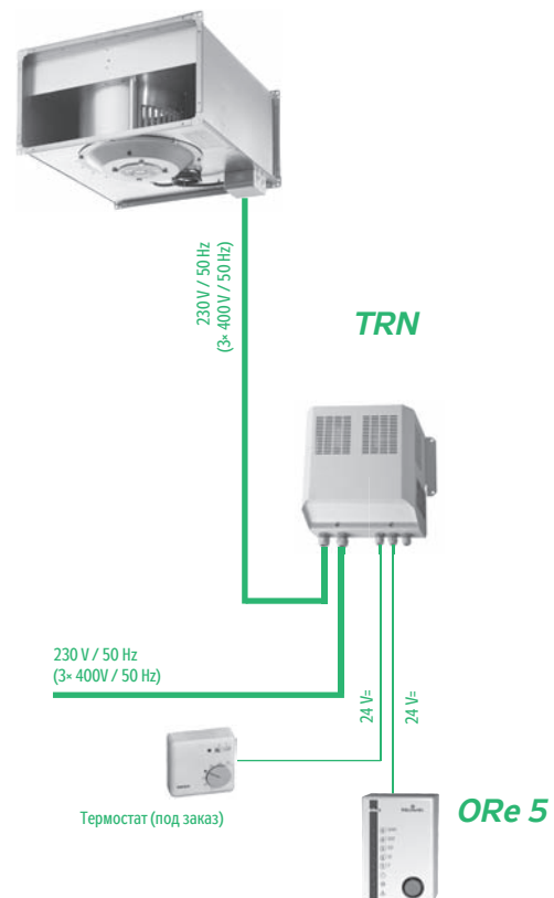
РИС. 8 – ПОДКЛЮЧЕНИЕ ВЕНТИЛЯТОРА
