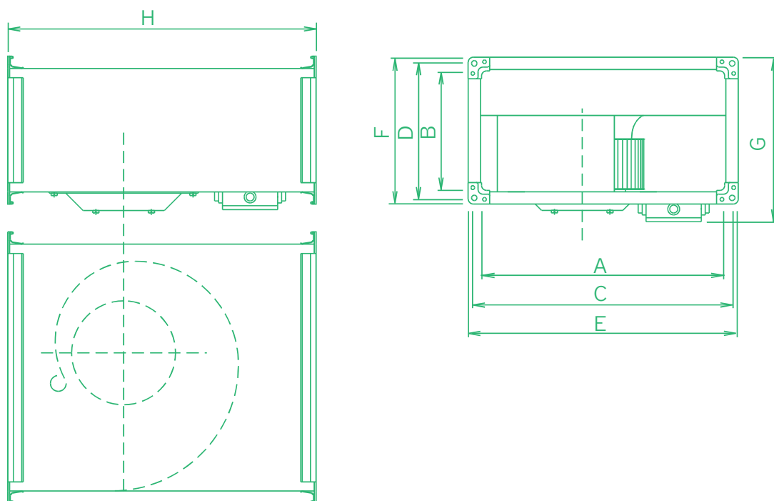
РИС. 5 – РАЗМЕРЫ ВЕНТИЛЯТОРОВ RP EX
