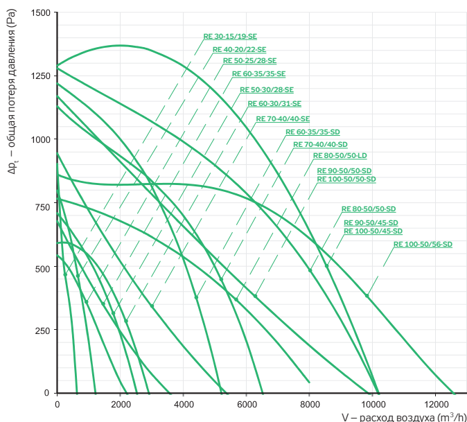
ГРАФИК 1 – ХАРАКТЕРИСТИКИ ВЕНТИЛЯТОРОВ RE
