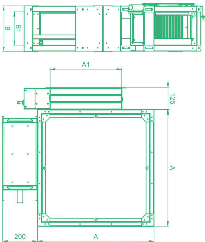
РИСУНОК 4 – РАЗМЕРЫ
