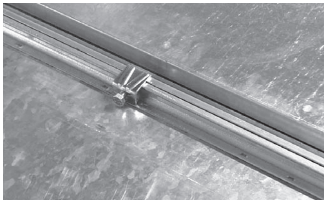
РИС. 11 – СОЕДИНЕНИЕ ПОСЕРЕДИНЕ СКОБОЙ
