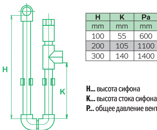
РИСУНОК 14 – ОТВОД КОНДЕНСАТА
