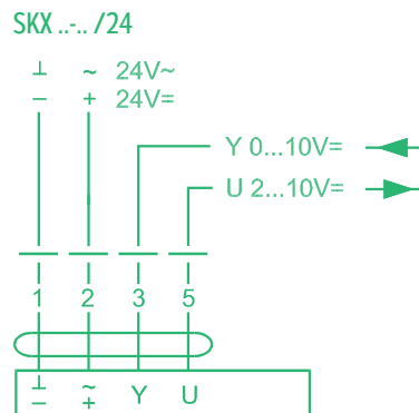
РИСУНОК 5 – ПОДКЛЮЧЕНИЕ СЕРВОПРИВОДА
