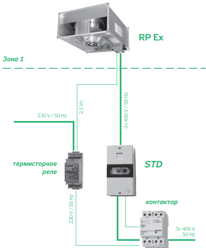
РИС. 11 – ПОДКЛЮЧЕНИЕ ВЕНТИЛЯТОРА
