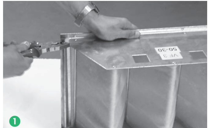
РИСУНОК 3 – ЗАМЕНА ТКАНИ ФИЛЬТРАЦИОННОГО ВКЛАДЫША
