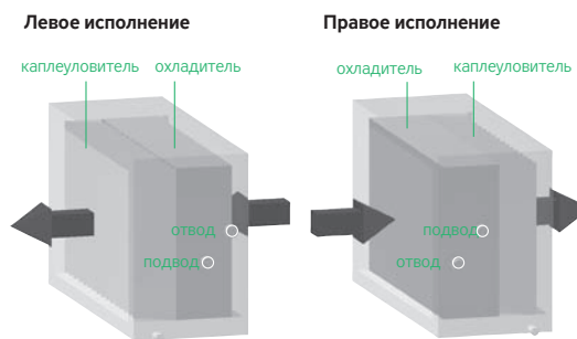
РИС. 7 - ПОДСОЕДИНЕНИЕ ОХЛАДИТЕЛЯ CHV
