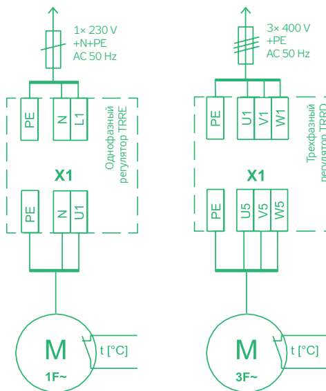
РИС. 33 – КЛЕММНАЯ СХЕМА РЕГУЛЯТОРОВ TRRE(D)
