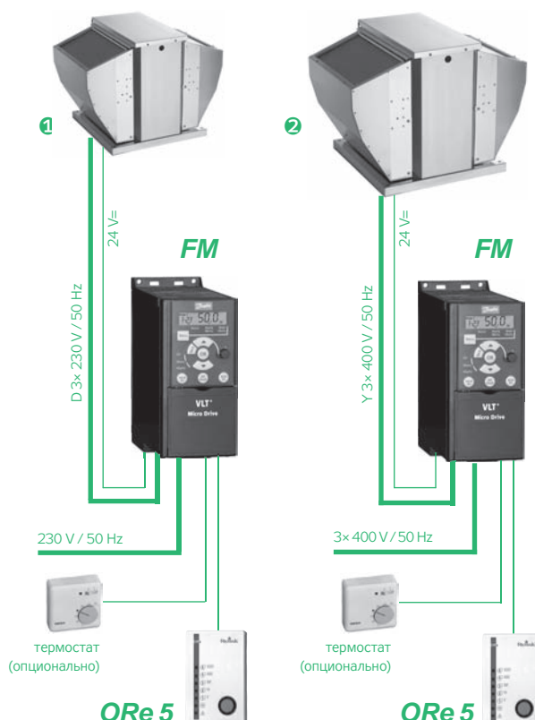
РИС.9 – ПОДКЛЮЧЕНИЕ ВЕНТИЛЯТОРА
