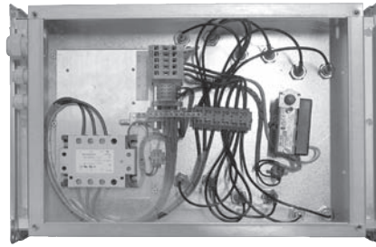
EOS... / 4-15, содержит один 3-фазный пускатель SSR. Вид внутри электрощита обогревателя EOS 50-30/15 при открытии крышки пускателей SSR.
