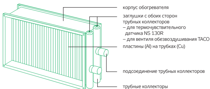
РИС. 2 – КОНСТРУКЦИЯ ОБОГРЕВАТЕЛЯ
