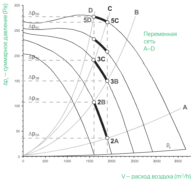
РИС. 3 – ХАРАКТЕРИСТИКА СЕТИ
