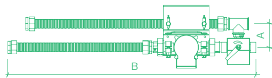
РИС. 3А – ОСНОВНАЯ КОМПОНОВКА
