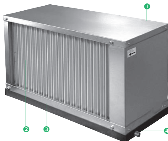
РИС. 3 – ОПИСАНИЕ ЧАСТЕЙ КАПЛЕУЛОВИТЕЛЯ
