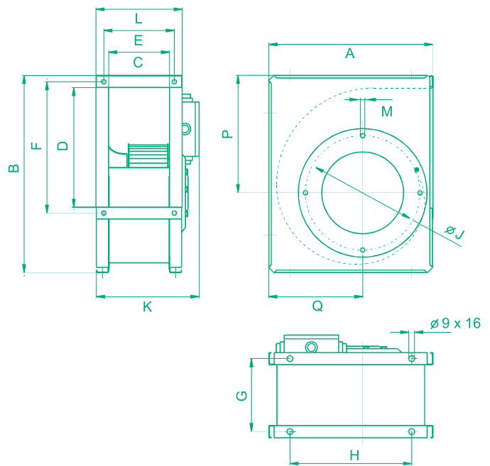
РИС. 2 – ОБОЗНАЧЕНИЕ РАЗМЕРОВ
