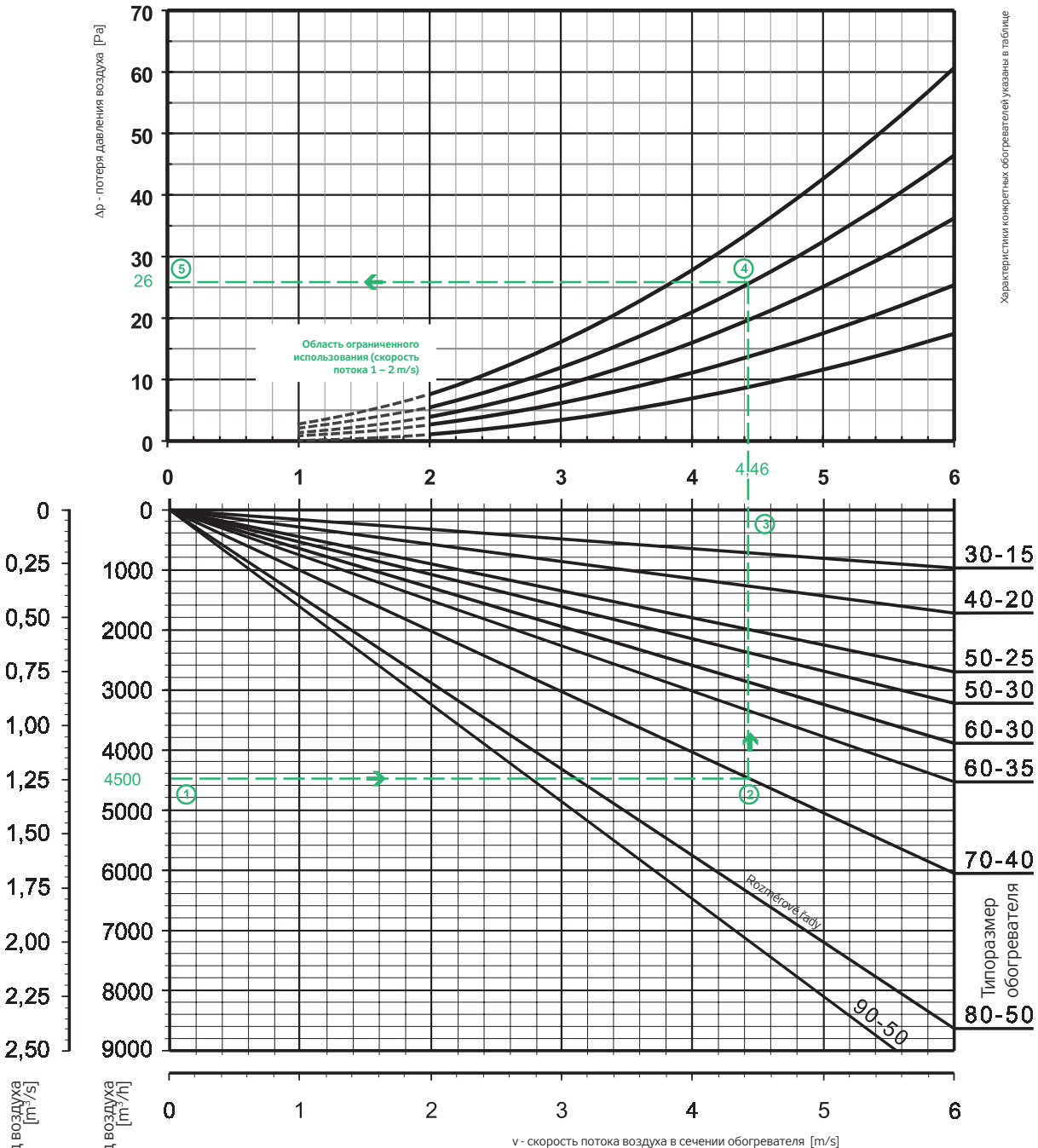
РИС. 5 – ПОТЕРИ ДАВЛЕНИЯ ОБОГРЕВАТЕЛЕЙ
