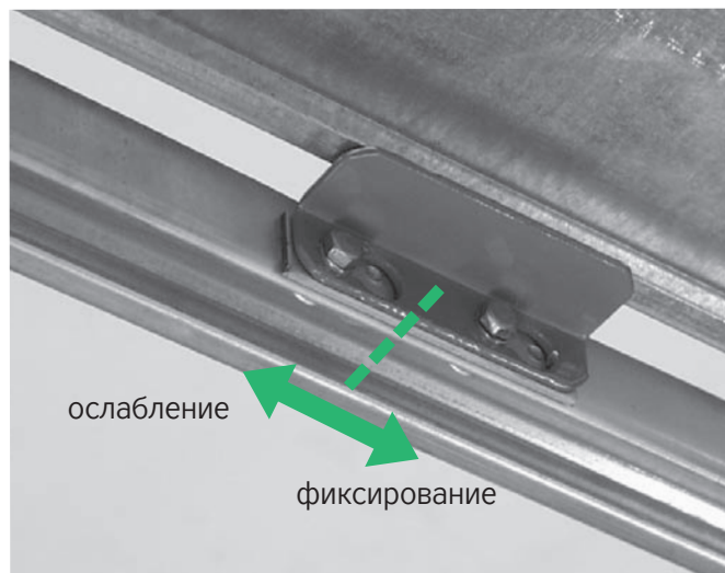
РИС. 13 – СОЕДИНЕНИЕ ПОСЕРЕДИНЕ СКОБОЙ
