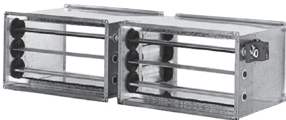
РИСУНОК 3 – СМЕСИТЕЛЬНАЯ КАМЕРА SKX С СЕРВОПРИВОДОМ NM 24A-SR
