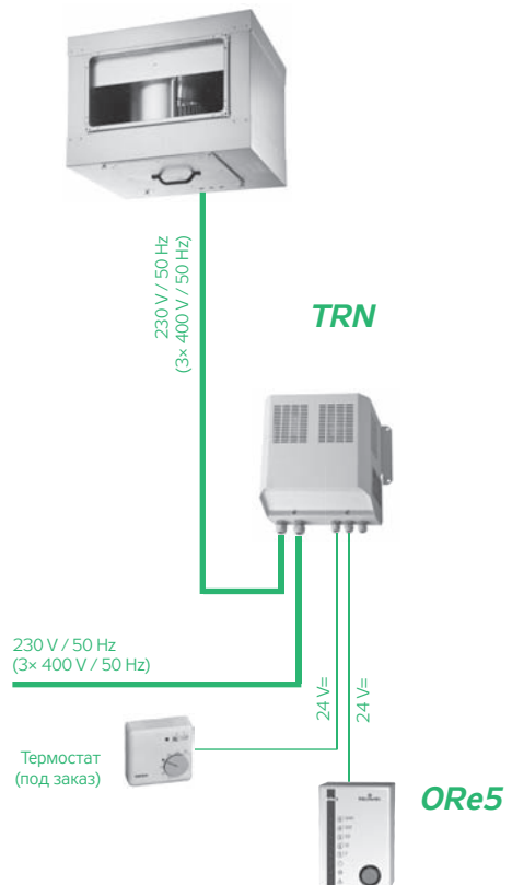
РИС. 7 – ПОДКЛЮЧЕНИЕ ВЕНТИЛЯТОРА
