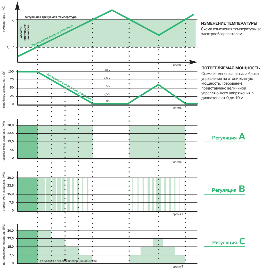
РИС. 8 – СХЕМАТИЧЕСКАЯ МОДЕЛЬ ВКЛЮЧЕНИЯ (РЕГУЛЯЦИИ) В ЗАВИСИМОСТИ ОТ ИЗМЕНЕНИЯ ТЕМПЕРАТУРЫ 4)
