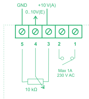
РИС. 41 – ПОДКЛЮЧЕНИЕ ОРР (IP 54)
