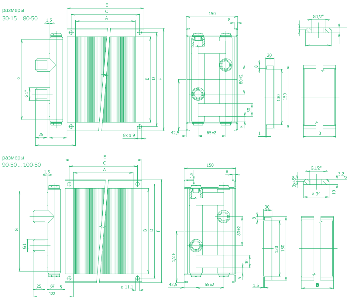
РИС. 5 – РАЗМЕРЫ ВОДЯНЫХ ОБОГРЕВАТЕЛЕЙ VO (СМ. ТАБЛИЦА 1)
