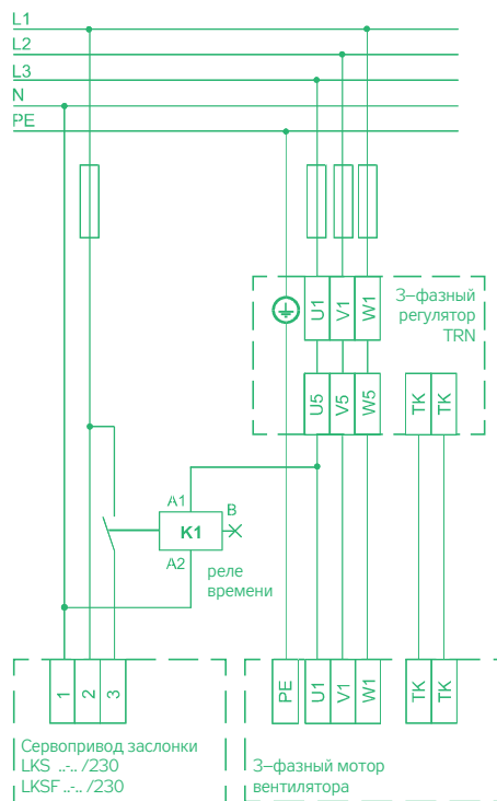
РИС. 20 – СХЕМА ПОДКЛЮЧЕНИЯ ЗАСЛОНКИ LKS, LKSF
