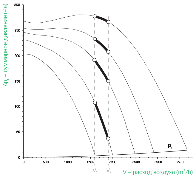
РИС. 2 – РАБОЧАЯ ХАРАКТЕРИСТИКА ВЕНТИЛЯТОРА
