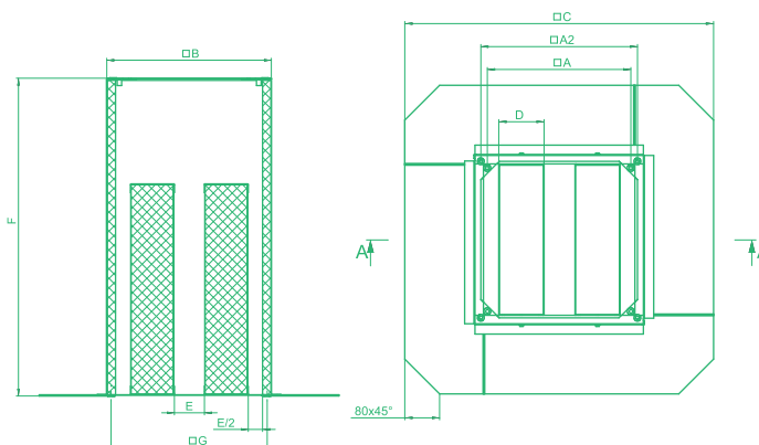
РИС.15 – РАЗМЕРЫ ПОДСТАВОК NDH
