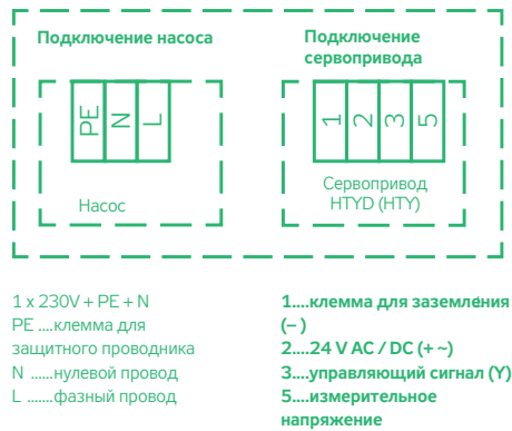
РИС. 8 – СХЕМА ПОДКЛЮЧЕНИЯ СМЕСИТЕЛЬНОГО УЗЛА
