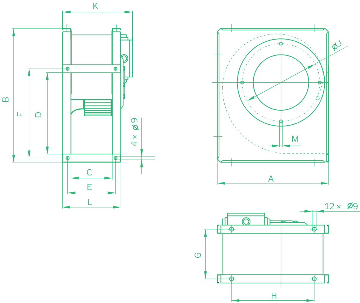
РИС. 5 – РАЗМЕРЫ ВЕНТИЛЯТОРОВ RP EX
