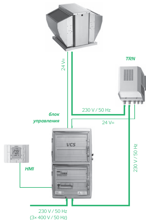
РИС.11 – ПОДКЛЮЧЕНИЕ ВЕНТИЛЯТОРА
