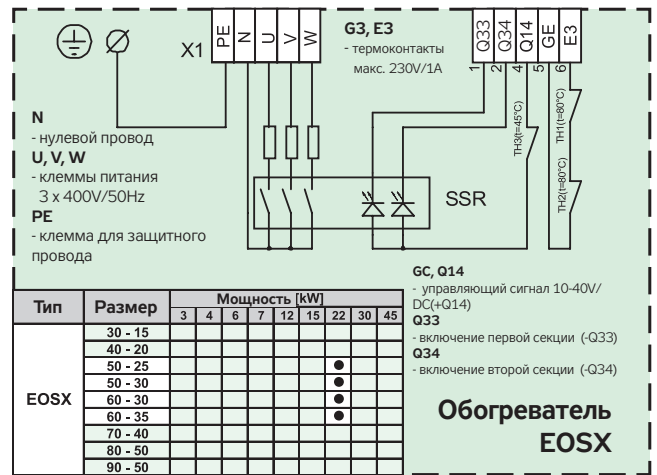
РИС. 22 – СХЕМА ПОДКЛЮЧЕНИЯ ОБОГРЕВ. EOSX
