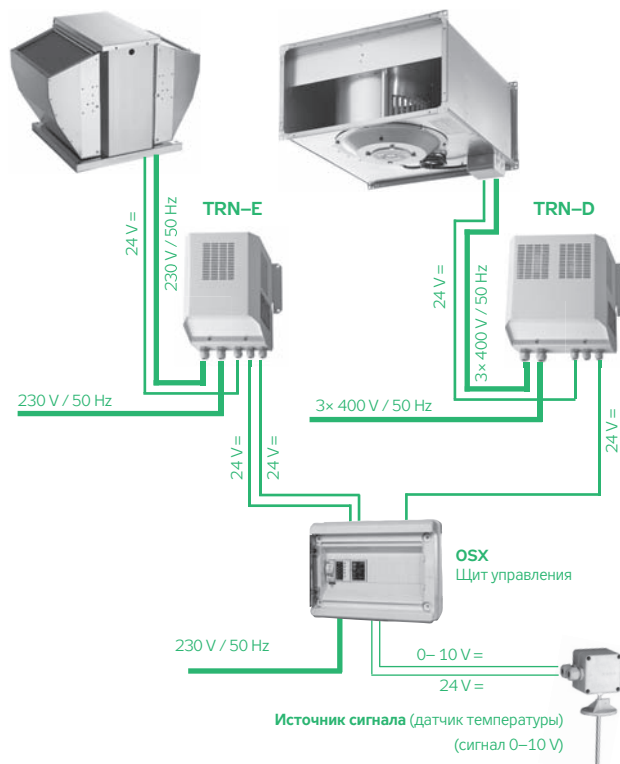
РИС. 24 – ПОДКЛЮЧЕНИЕ РЕГУЛЯТОРОВ
