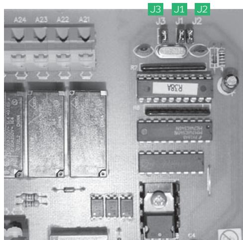
РИС. 18 – ОПИСАНИЕ СОЕДИНИТЕЛЕЙ
