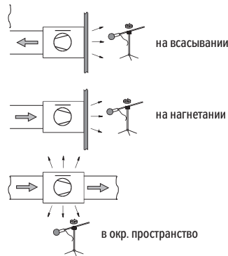
РИС. 4 – ОРИЕНТИРОВКА ВЕНТИЛЯТОРА ПО ОТНОШЕНИЮ К ПРОСТРАНСТВУ
