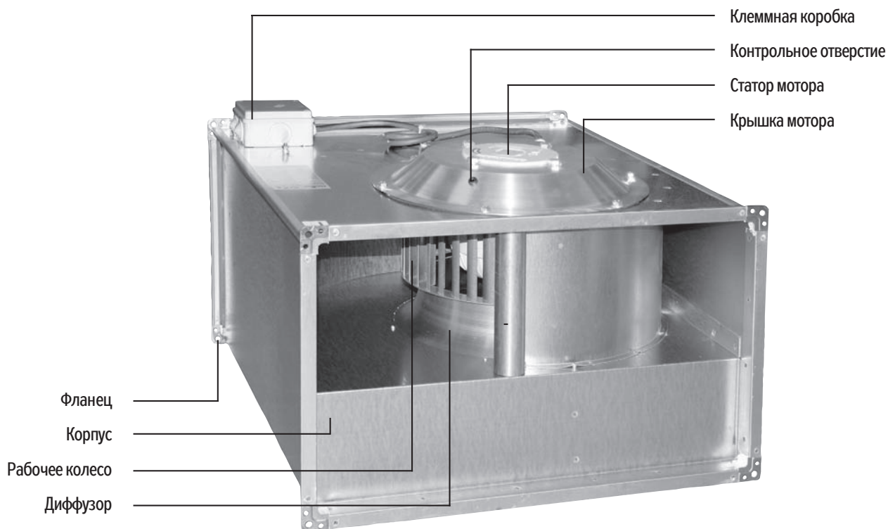
РИС. 3 – ВЕНТИЛЯТОР RP
