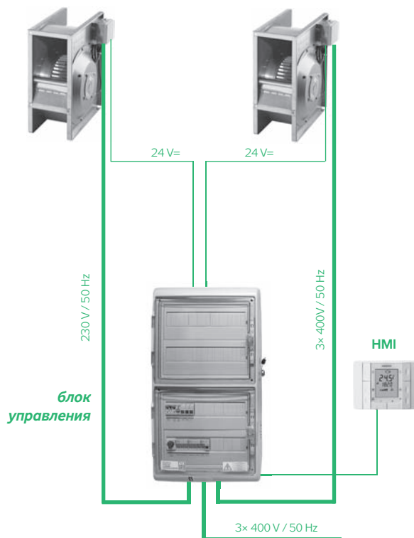
РИС. 7 – ПОДКЛЮЧЕНИЕ ВЕНТИЛЯТОРА
