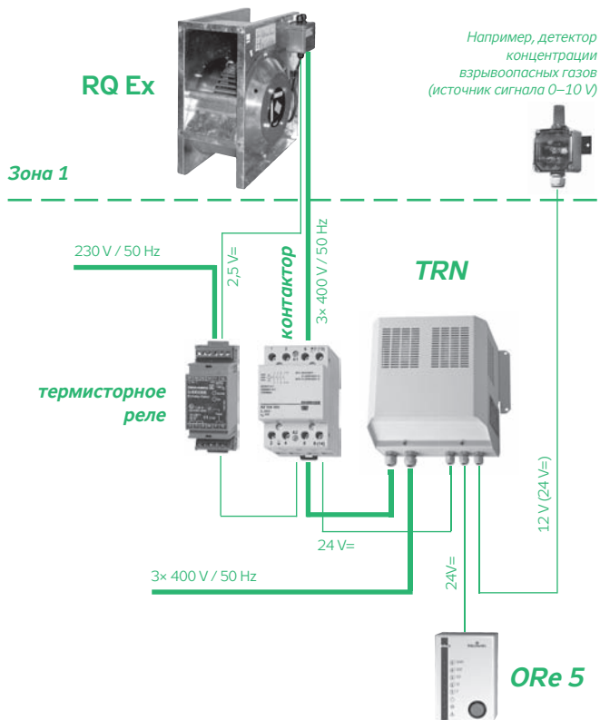
РИС. 12 – ПОДКЛЮЧЕНИЕ ВЕНТИЛЯТОРА
