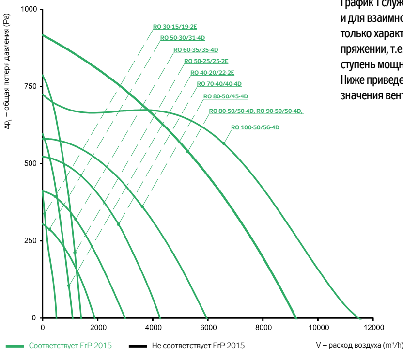
ГРАФИК 1 – ХАРАКТЕРИСТИКИ ВЕНТИЛЯТОРОВ RO ДЛЯ БЫСТРОГО ПОДБОРА
