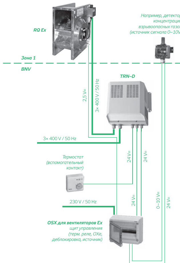
РИС. 15 – ПОДКЛЮЧЕНИЕ ВЕНТИЛЯТОРА
