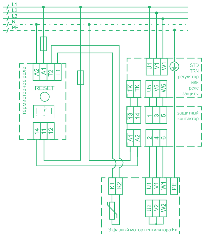
РИС. 7 – ПРИМЕР ПОДКЛЮЧЕНИЯ ТЕРМИСТОРНОГО РЕЛЕ
