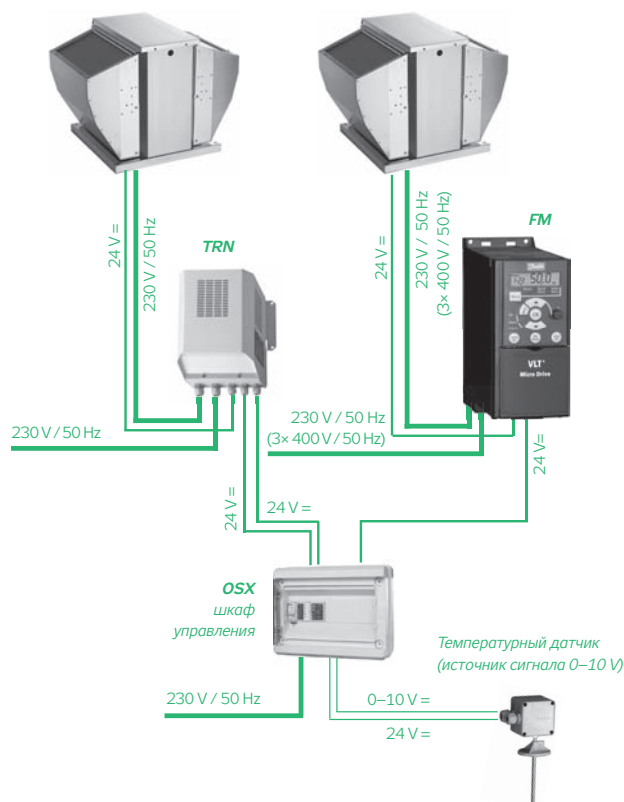
РИС.13 – ПОДКЛЮЧЕНИЕ ВЕНТИЛЯТОРА
