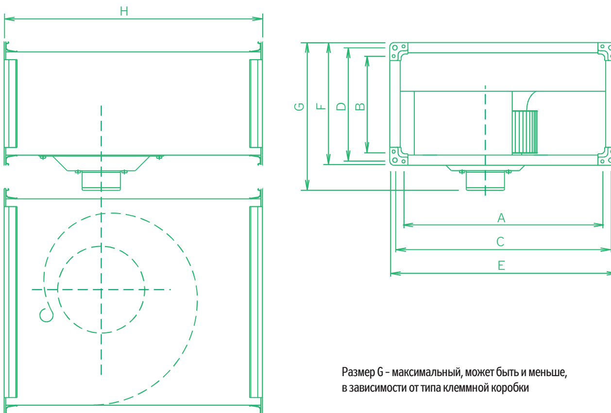
РИС. 5 – ОБОЗНАЧЕНИЕ РАЗМЕРОВ
