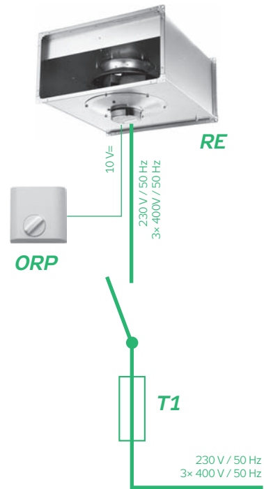
РИС. 21 – ПОДКЛЮЧЕНИЕ КОМАНДОАППАРАТА
