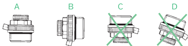
РИС. 9 – ПОЛОЖЕНИЯ ВЕНТИЛЯ ТАСО
