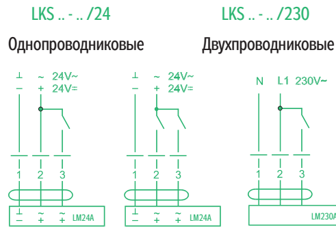
РИСУНОК 4 – ПОДКЛЮЧЕНИЕ СЕРВОПРИВОДА
