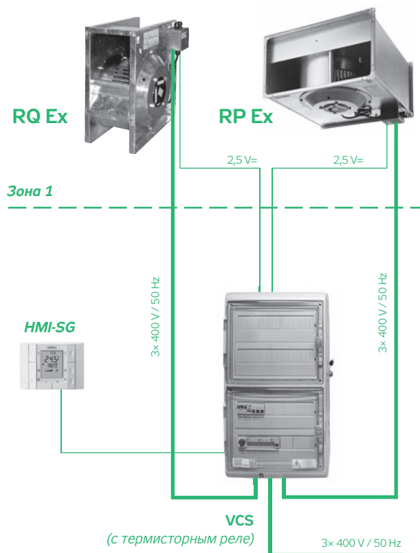
РИС. 13 – ПОДКЛЮЧЕНИЕ ВЕНТИЛЯТОРА
